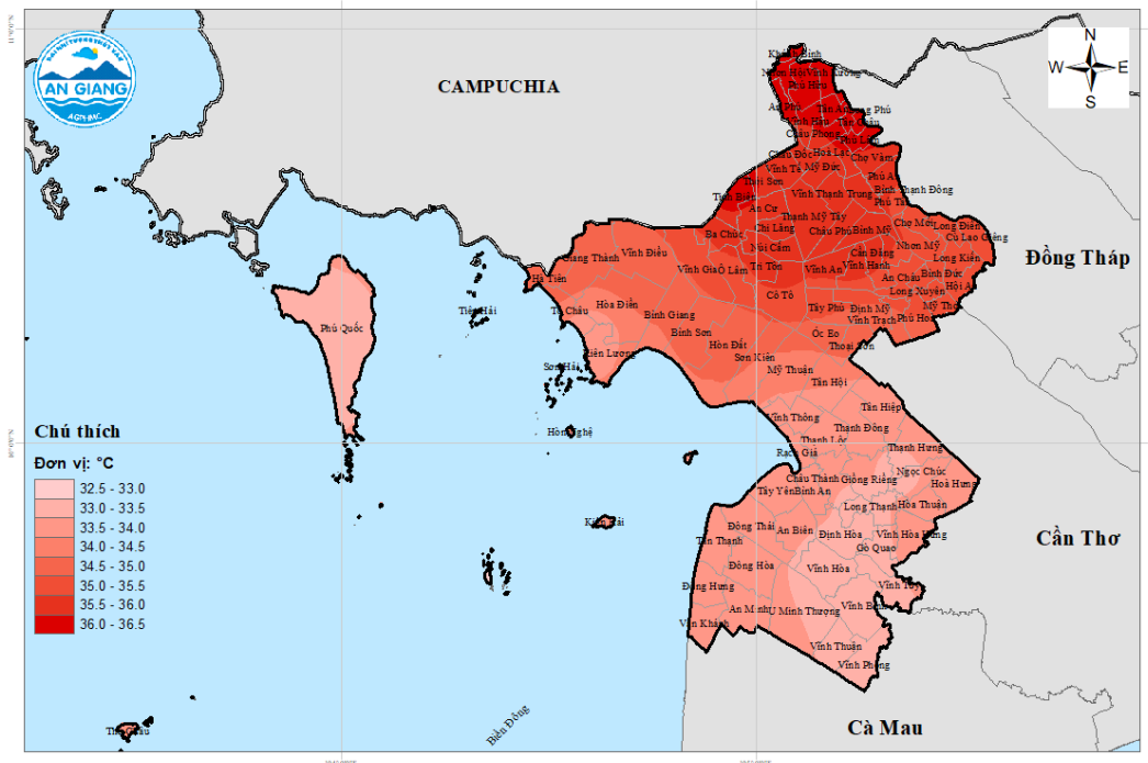
BẢN ĐỒ DỰ BÁO NHIỆT ĐỘ CAO NHẤT TRONG 24 GIỜ NGÀY 02/4/2026 TỈNH AN GIANG
