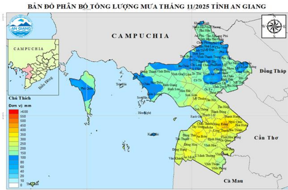
Hình 2: Bản đồ phân bố tổng lượng mưa tháng 11/2025 tỉnh An Giang
