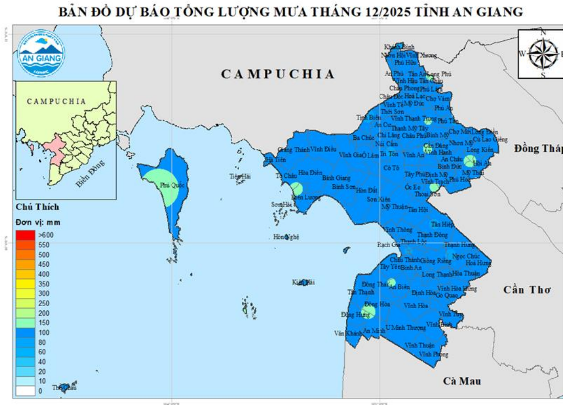
Hình 4: Bản đồ dự báo tổng lượng mưa tháng 12/2025 tỉnh An Giang
