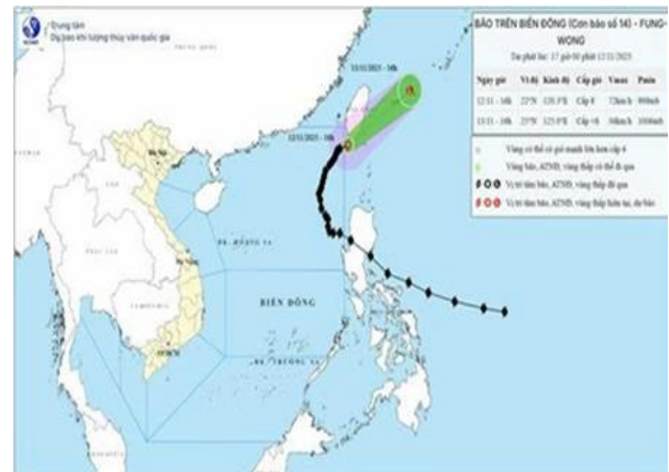
Quỹ đạo của Bão số 14
