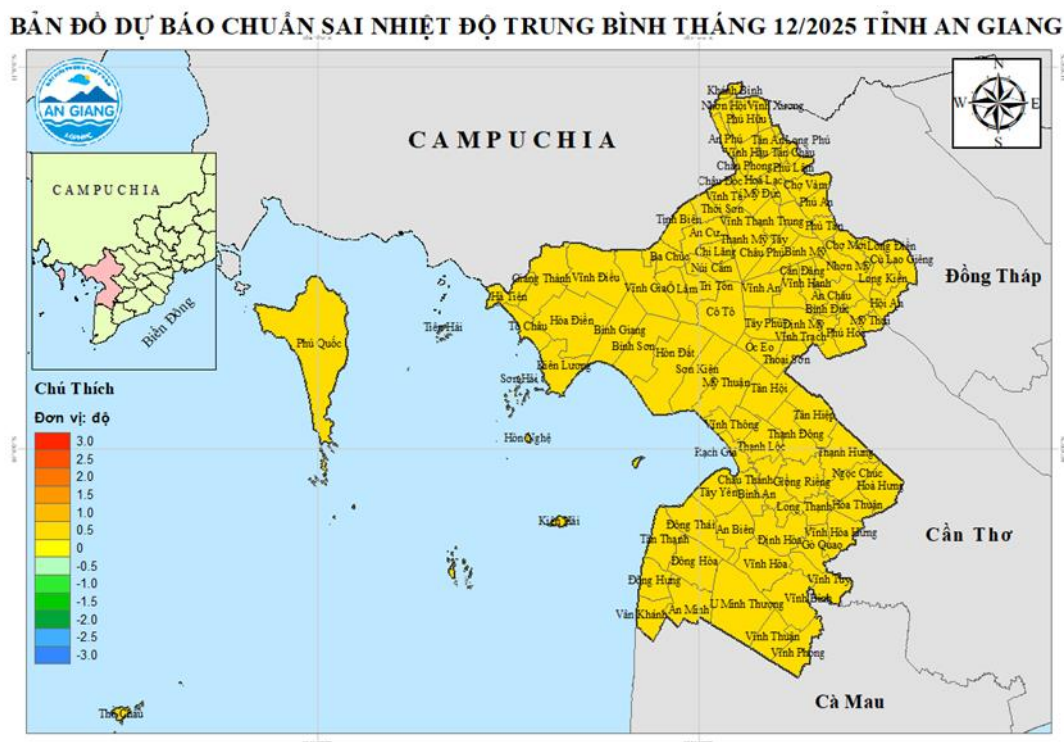
Hình 3: Bản đồ dự báo chuẩn sai nhiệt độ trung bình tháng 12/2025 tỉnh An Giang
