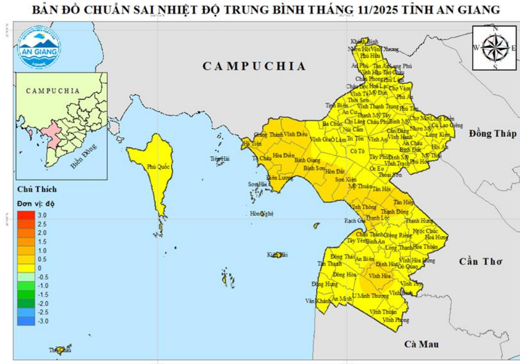
Hình 1: Bản đồ chuẩn sai nhiệt độ trung bình tháng 11/2025 tỉnh An Giang
