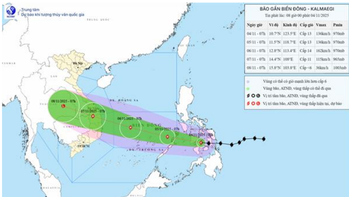
Hình 1: Bản đồ dự báo quỹ đạo và cường độ bão KALMAEGI phát lúc 08h00 ngày 04/11/2025
