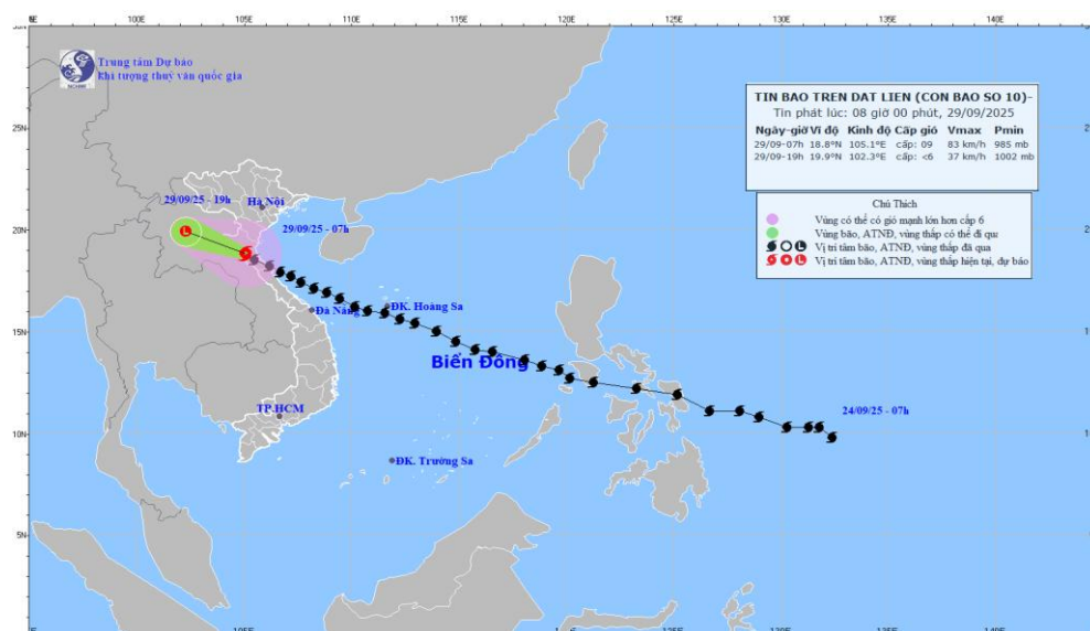
Hình1. Bản đồ dự báo quỹ đạo và cường độ bão số 10 phát lúc 08h00 ngày 29/9/2025
