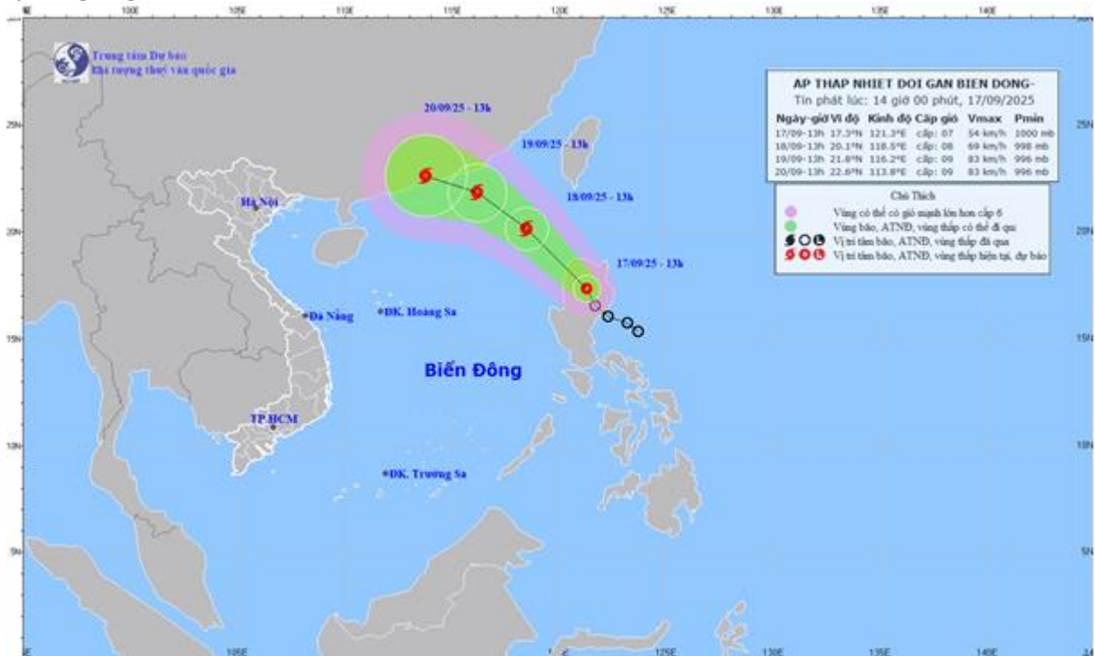
Hình 01. Bản đồ dự báo quỹ đạo và cường độ áp thấp nhiệt đới gần Biển Đông phát lúc 14h00 ngày 17/9/2025
