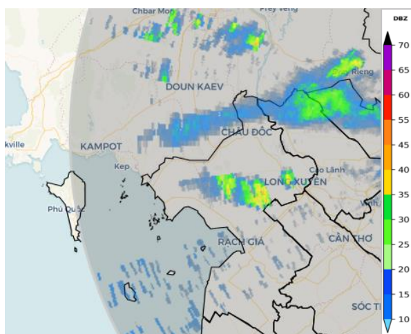
Ảnh Radar thời tiết tại An Giang
