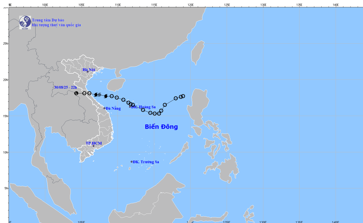
Hình 1. Bản đồ quỹ đạo bão số 6
