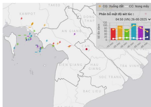
Ảnh định vị sét tại An Giang
