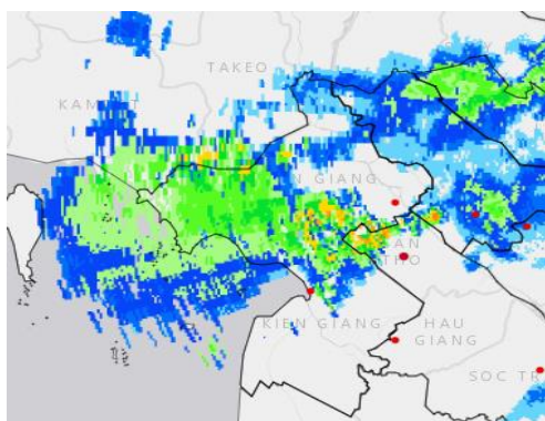
Ảnh Radar thời tiết tại An Giang
